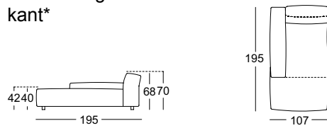
Hoekaanbouwelement*
