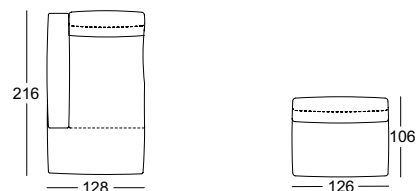
Extra diepte-Afsluitdeelaanbouwbank*
